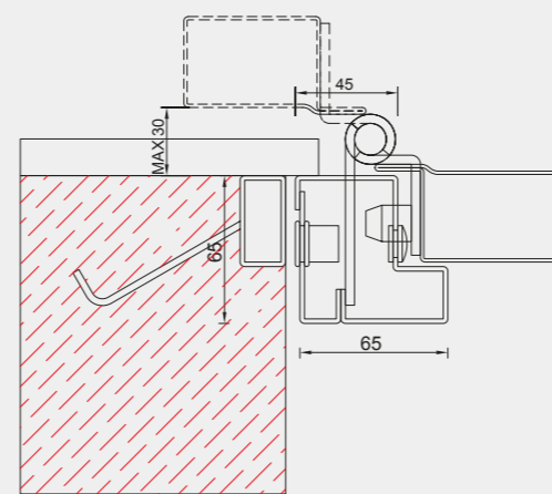
Telaio per persiane modello Onda
