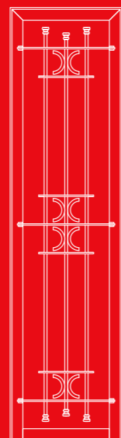
Mod. 3 - tondo diam. 14 - piatto 30x8 + mezzi cerchi
