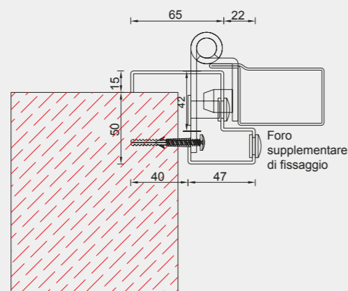
Telaio standard con fori supplementari di fissaggio per persiane, grate e scuroni apribili
