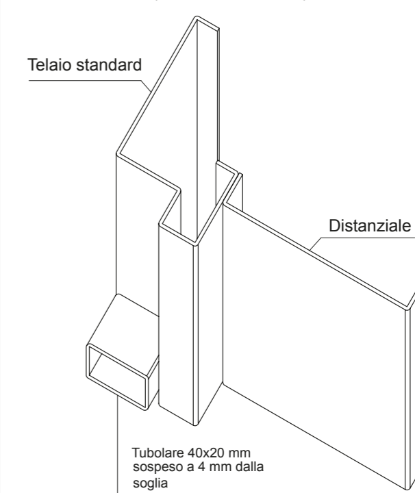
Telaio standard con distanziale da 80 - 100 - 120 mm per grate, persiane e scuroni apribili
