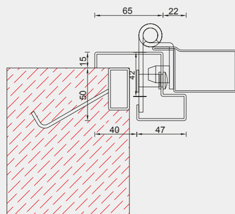
Telaio standard per persiane, grate e scuroni apribili
