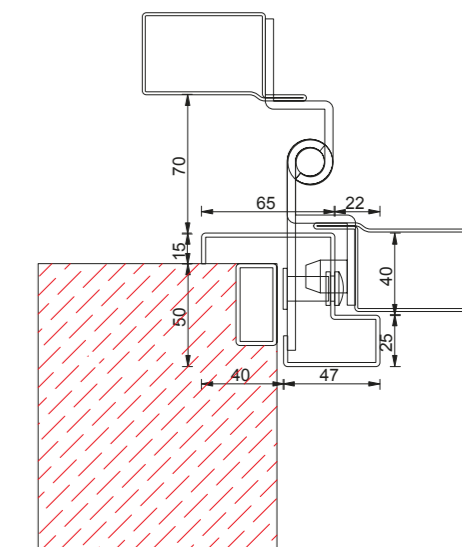
Telaio con cerniera a collo alto
