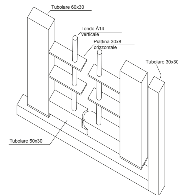
Particolare della grata a snodo
