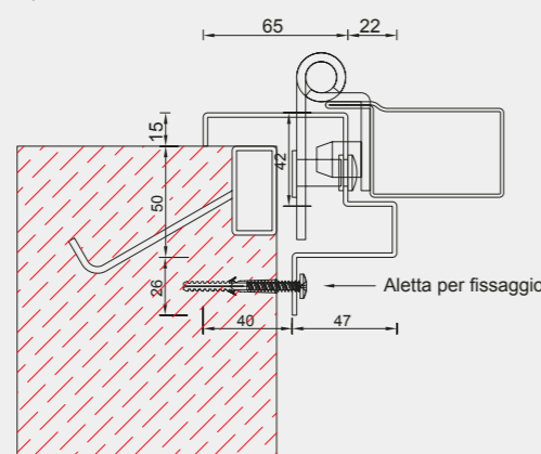
Telaio standard con fori supplementari di fissaggio per persiane, grate e scuroni apribili
