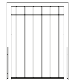
Mod. 7 piatto 40x8 orizzontale e tondo diam. 16 mm verticale
