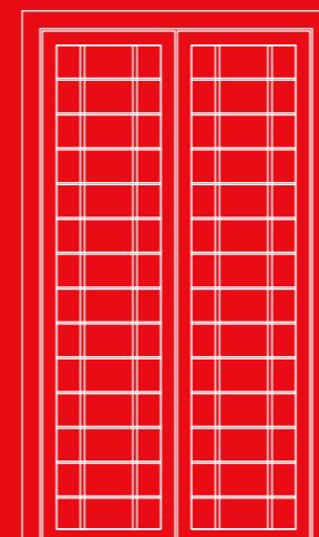
Mod. 5 piatto 40x8 orizzontale e tondo diam. 16 mm verticale + borchie e semi borchie
